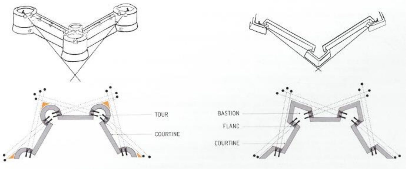
Représentation schématique du principe de flanquement L'angle mort devant la tour médiévale (en jaune), le flanquement réciproque parfait devant le bastion pentagonal
